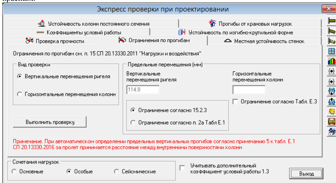
Рис. 7. 9 Экспресс-проверка прочности
