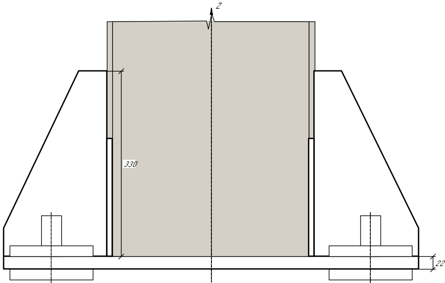
Рис. 1. К расчету прочности сварных швов
