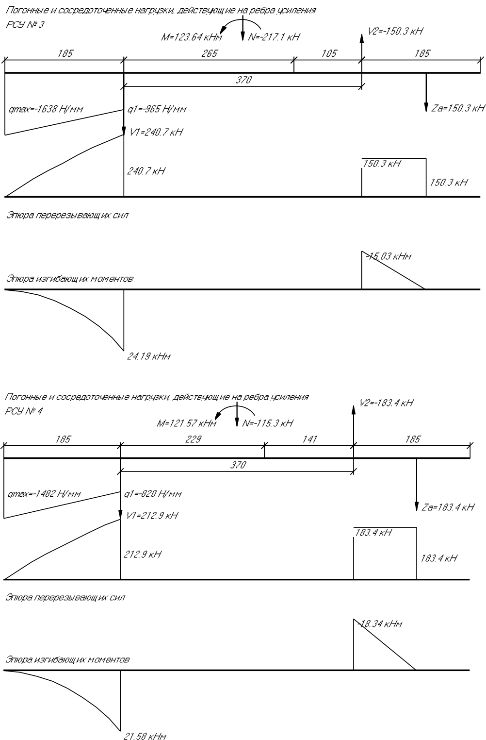
Рис. 2. Расчетная схема для ребра по оси X
