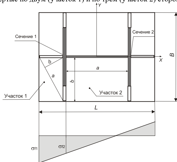
Рис. 3. Схема к расчету опорной плиты колонны, моментно опирающейся на фундамент, с ребрами усиления
