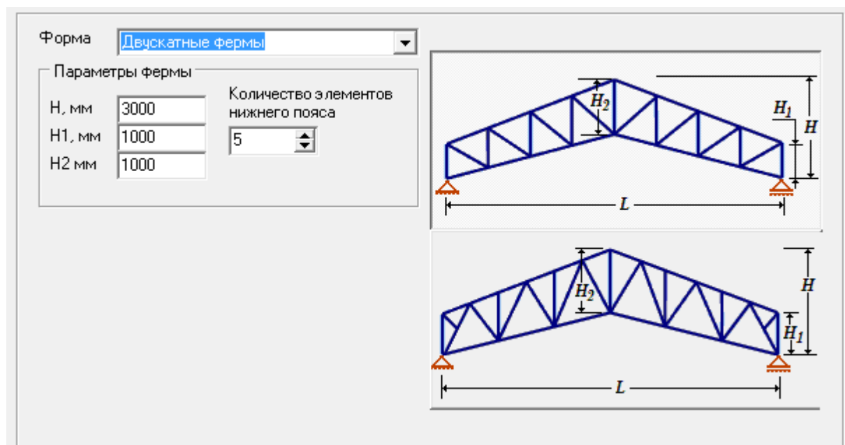
Рис. 1. 12. Двускатные фермы
