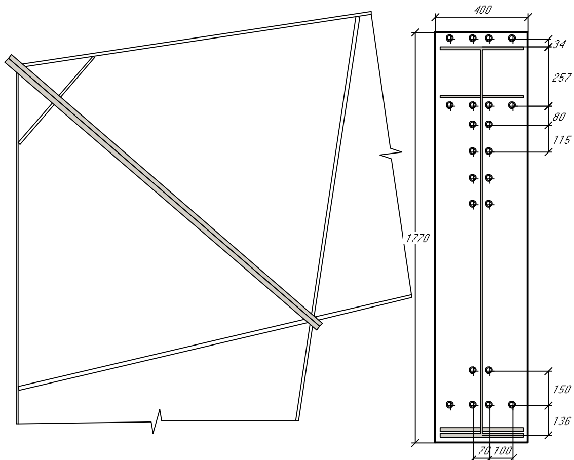
Рис. 3. Эскиз фланцевого узла
