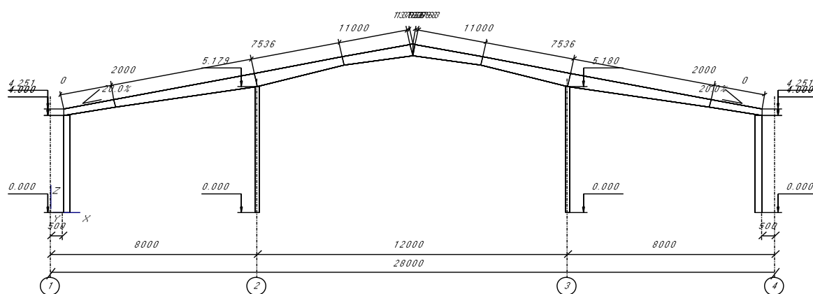
Рис. 1.5. Многопролетная одноэтажная рама жестким сопряжением колонн с фундаментом и шарнирным опиранием ригеля на колонны.
