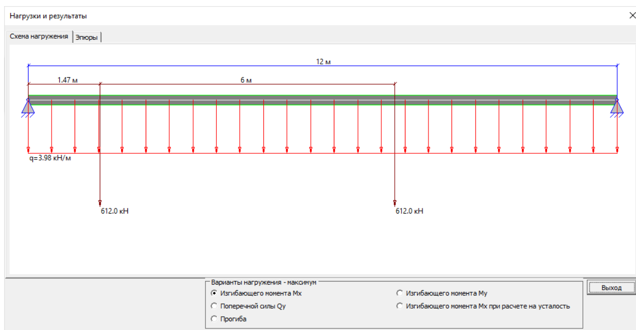
Рис. 17.5. Схема нагружения балки при действии максимального изгибающего момента
