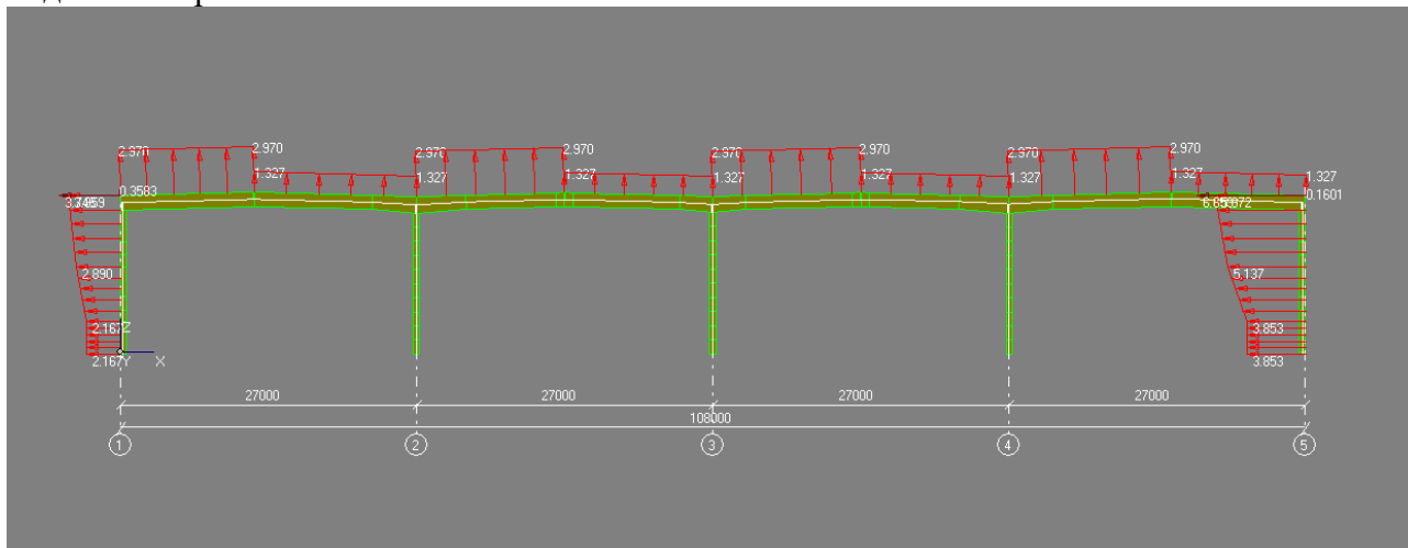
Рис. 1.6. Многопролетная многоконьковая одноэтажная рама жестким сопряжением колонн с фундаментом и шарнирным опиранием ригеля на колонны
