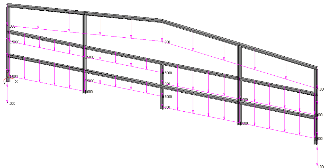
Рис. 1.8. Одноконьковая, многопролетная, многоуровневая рама
