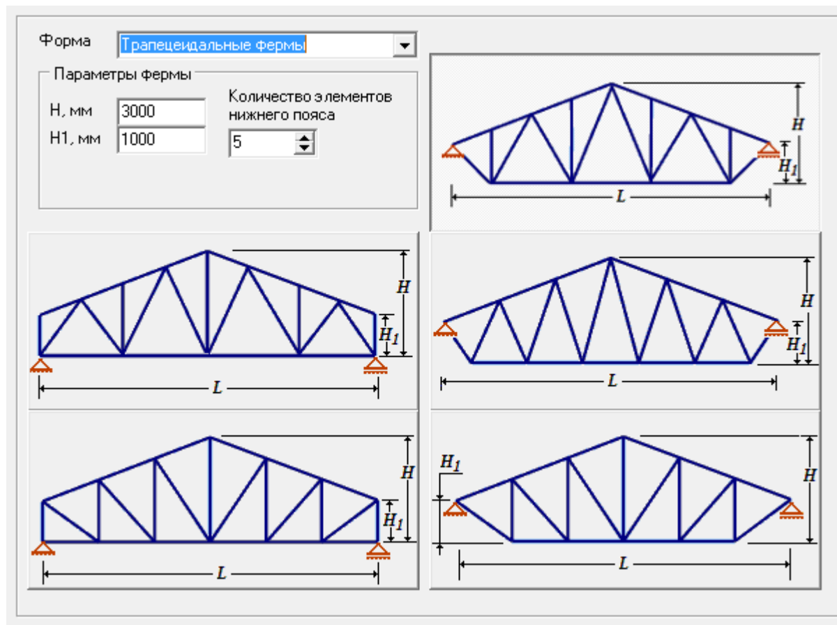
Рис. 1. 10. Трапециевидальные фермы
